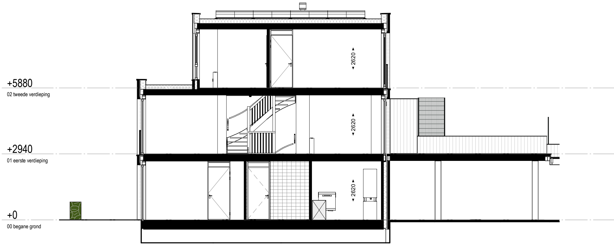
Dwarsdoorsnede 1 : 100
