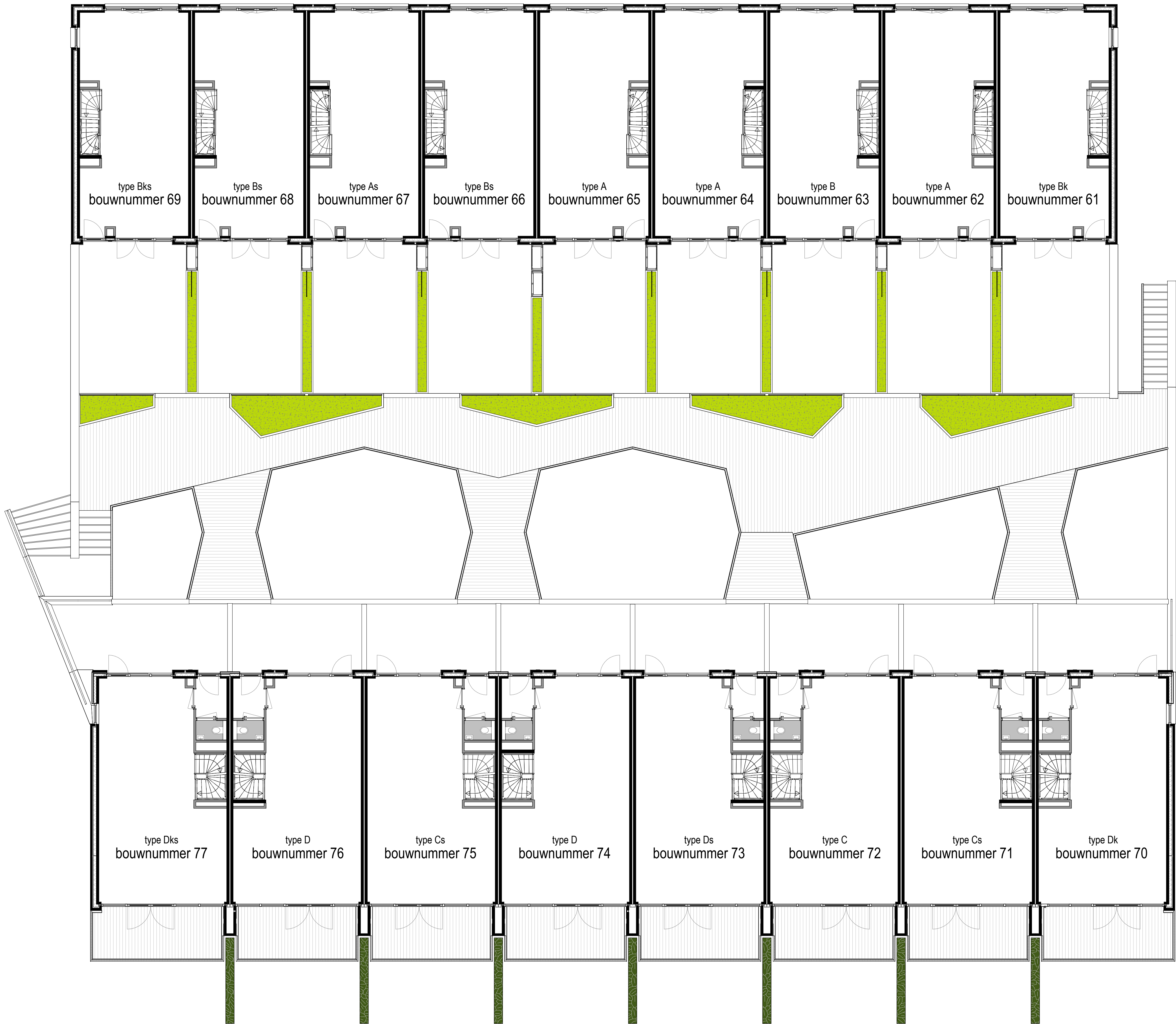
Eerste verdieping blok F + G 1 : 100
