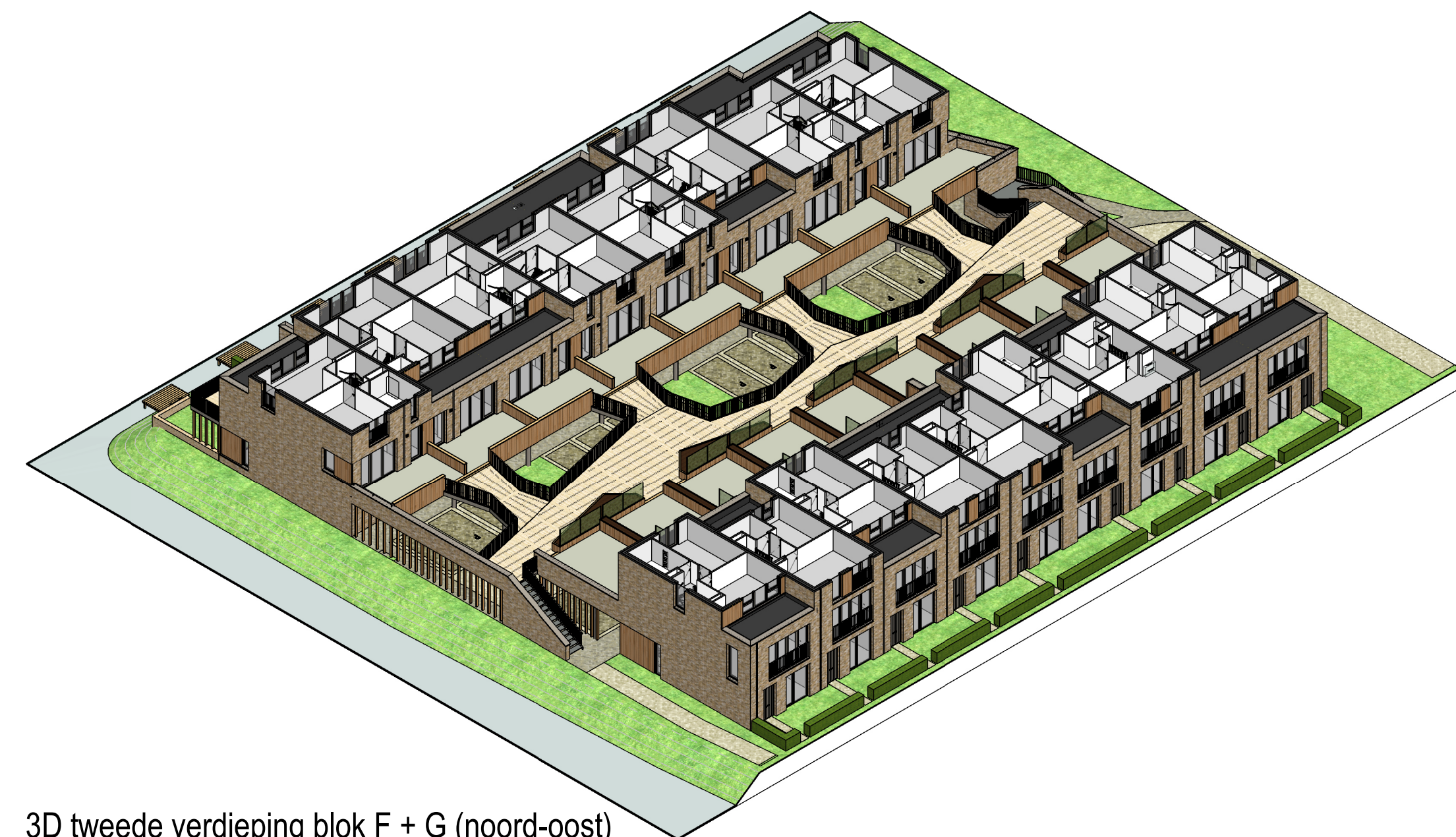
3D tweede verdieping blok F + G (noord-oost)
