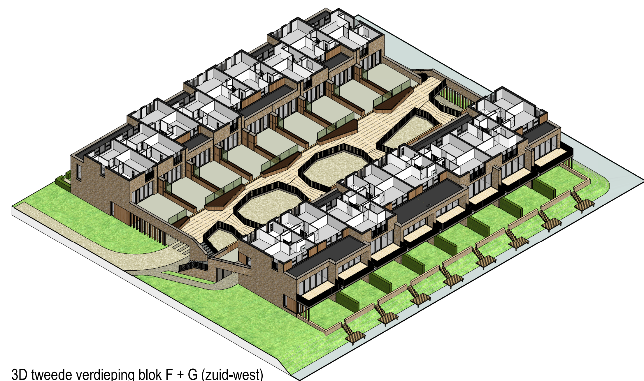
3D tweede verdieping blok F + G (zuid-west)
