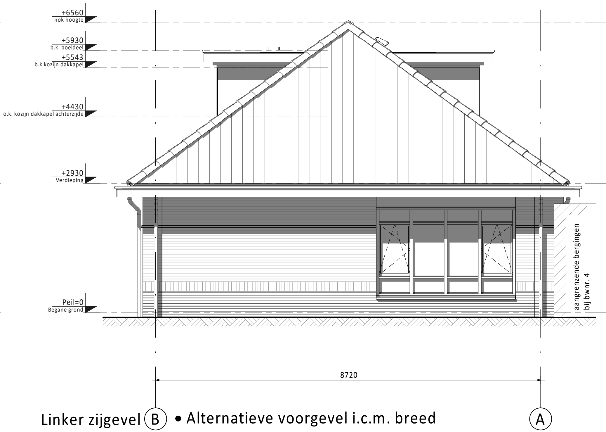
Linker zijgevel (B) • Alternatieve voorgevel i.c.m. breed kozijn zijgevel (standaard en alleen mogelijk bij bwnr. 04 ) • Dakkapel achterzijde (niet mogelijk bij bwnrs. 07 t/m 10) (A)
