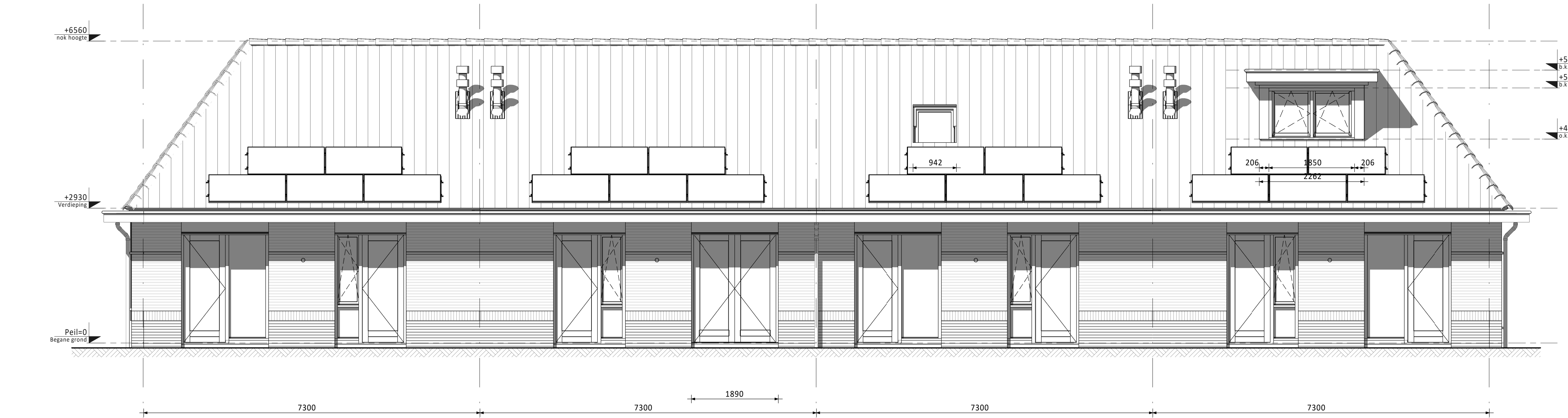
Achtergevel (as) • Basis achtergevel (as) • Dubbele deuren achtergevel i.p.v. enkele deur (as) • Dakraam achterzijde (as) • Dakkapel achterzijde (niet mogelijk bij bwnrs. 07 t/m 10) (as)
