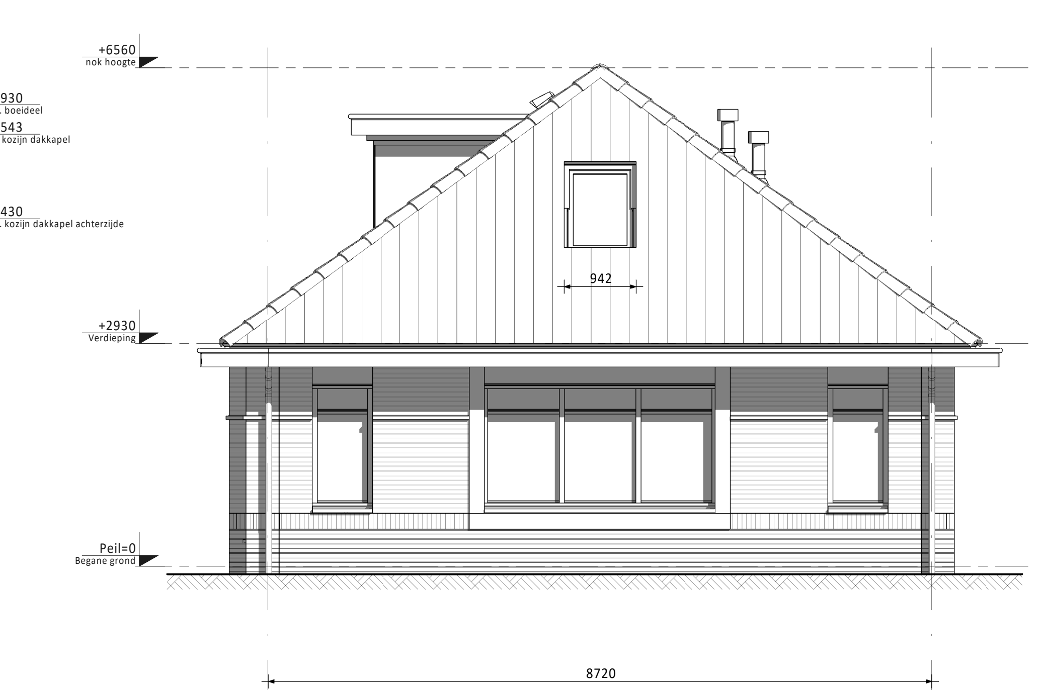
Rechter zijgevel (A) • Alternatieve zijgevel (standaard en alleen mogelijk bij bwnrs. 01 en 10) • Dakraam kopgevelzijde (B)
